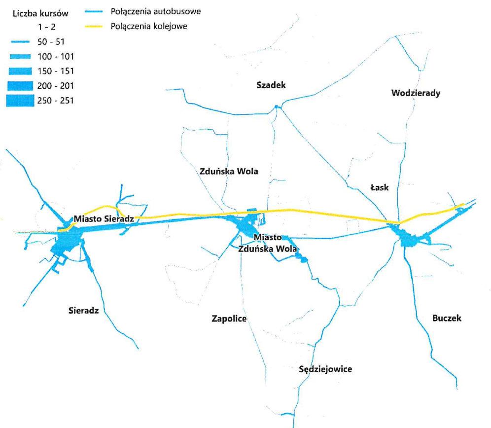
Rysunek 2.9 Liczba kursów komunikacji na obszarze MOF
